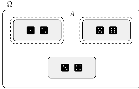
Figura 2: A \sigma -álgebra do Exemplo 5: os três blocos formam uma partição de \Omega , e cada evento é uma união de blocos. Em destaque, o evento A = \{\blacksquare, \square, \blacksquare, \square\} .
