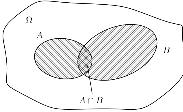
Figura 1: Diagrama de Venn que ilustra a identidade \mathbb{P}(A \cup B) = \mathbb{P}(A) + \mathbb{P}(B) - \mathbb{P}(A \cap B) .
