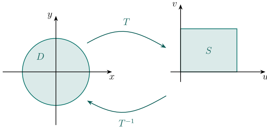
Figura 2: Representação esquemática de uma bijeção T : D \rightarrow S entre duas regiões do plano e de sua inversa T^{-1} : S \rightarrow D .
