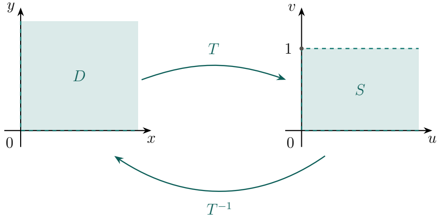
Figura 4: A transformação T(x, y) = \left(x + y, \frac{x}{x + y}\right) .
