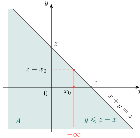
Figura 1: O semiplano A = \{(x, y) : x + y \leq z\} , sombreado, inclui a reta x + y = z e se estende além da janela desenhada. Para cada x = x_0 , a seção vertical indicada em vermelho é dada por -\infty < y \leq z - x_0 .
