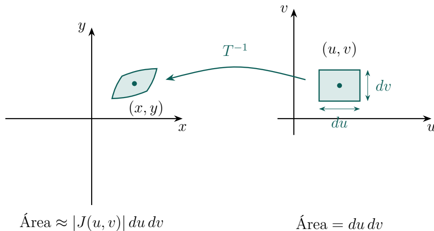
Figura 3: Dilatação local de área pela aplicação inversa T^{-1} . O quadrilátero de lados curvos representa a imagem do pequeno retângulo; a razão entre as áreas tende a |J(u, v)| quando o retângulo encolhe em torno de (u, v) .
