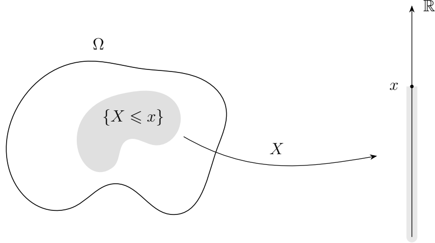
Figura 1: O evento \{X \leq x\} \equiv \{\omega \in \Omega : X(\omega) \leq x\}
