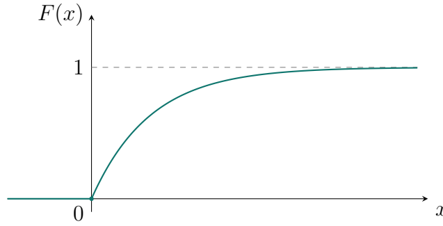
Figura 4: Função de distribuição exponencial com parâmetro \lambda . A função é identicamente nula em (-\infty, 0] e tende assintoticamente a 1 quando x \rightarrow +\infty .
