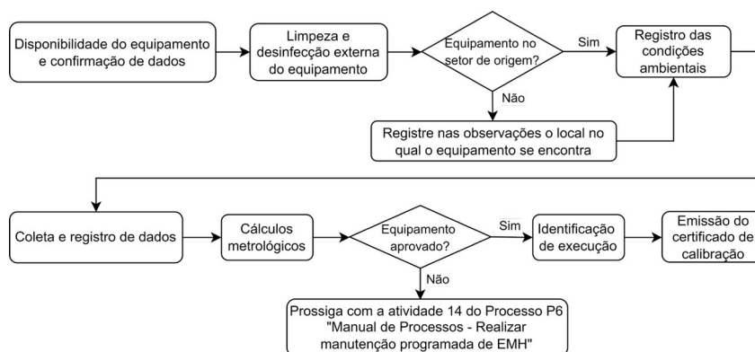
Figura 3 - Etapas de execução do procedimento de calibração de balança antropométrica adulto.
