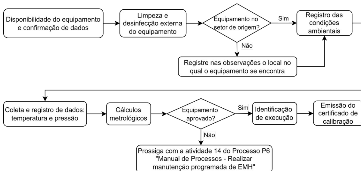
Figura 3 - Etapas de execução do procedimento de calibração em equipamentos do tipo autoclave vertical.
