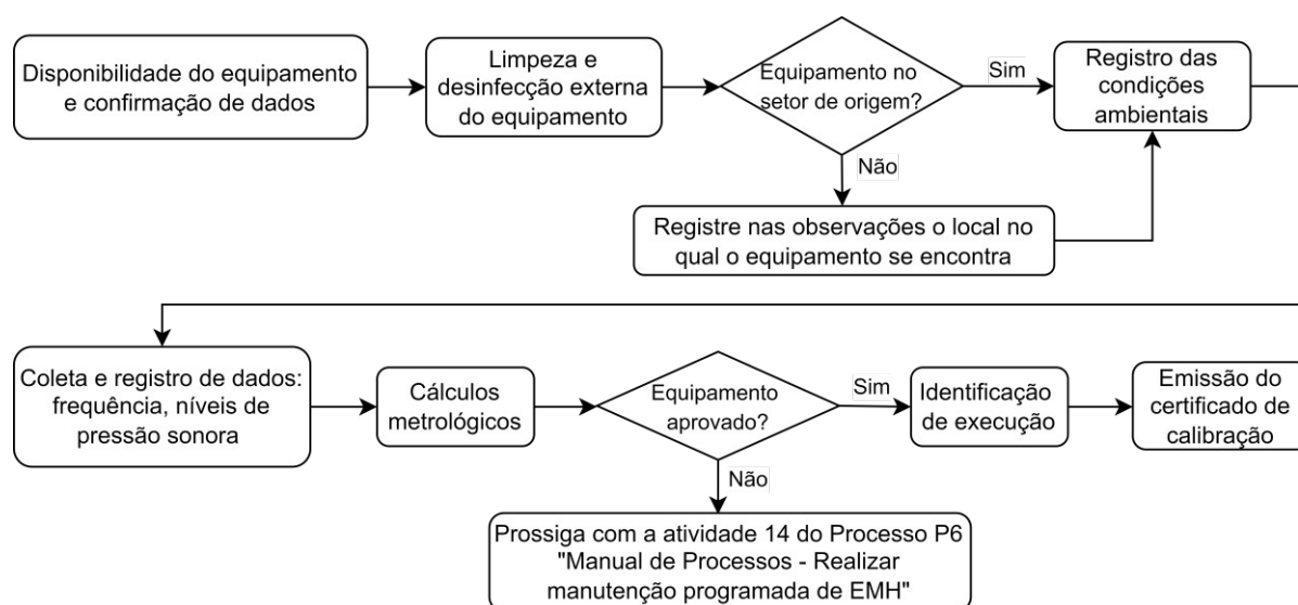
Figura 3 - Etapas de execução do procedimento de calibração de equipamento do sis triagem auditiva RN.
