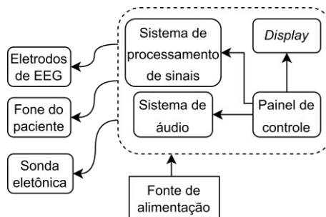
Figura 2 - Diagrama em blocos de um equipamento do tipo sis triagem auditiva RN.
