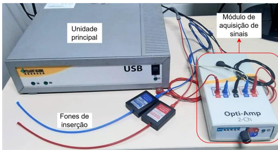
Figura 1 - Equipamento do tipo sis triagem auditiva RN.
