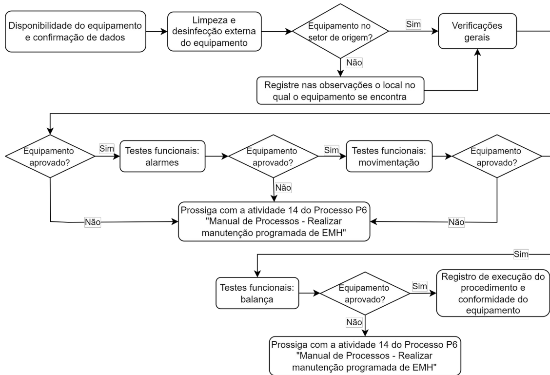
Figura 3 - Etapas de execução de procedimento de manutenção preventiva de equipamentos do tipo cama elétrica.
