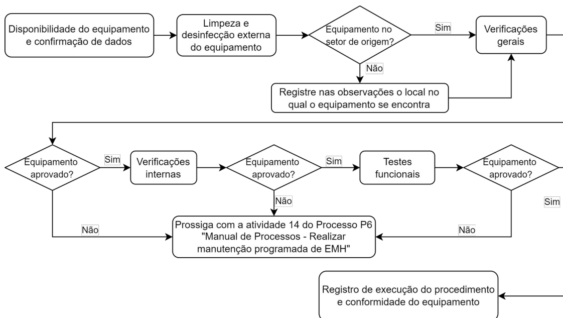
Figura 4 - Etapas de execução de procedimento de manutenção preventiva em equipamentos do tipo incubadora biológica.
