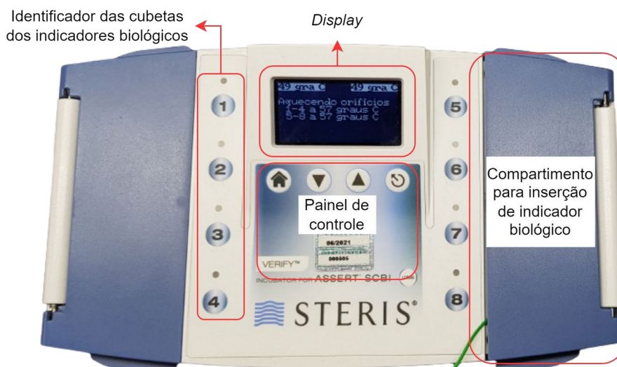
Figura 1 – Incubadora biológica.
