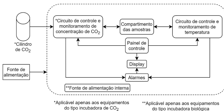
Figura 3 - Diagrama em blocos de um equipamento do tipo incubadora biológica.
