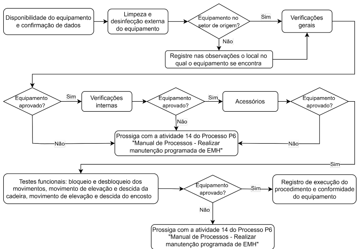
Figura 3 - Etapas de execução do procedimento de manutenção preventiva de equipamentos do tipo cadeira exame tratamento odontológico.
