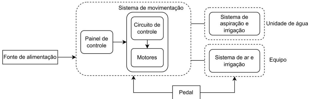
Figura 2 - Diagrama em blocos de equipamento do tipo cadeira exame tratamento odontológico.
