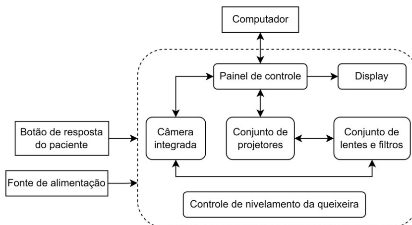
Figura 2 - Diagrama em blocos de equipamento do tipo campímetro.
