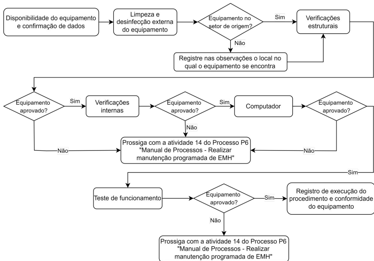
Figura 3 - Etapas de execução de procedimento de manutenção preventiva em equipamento do tipo campímetro.
