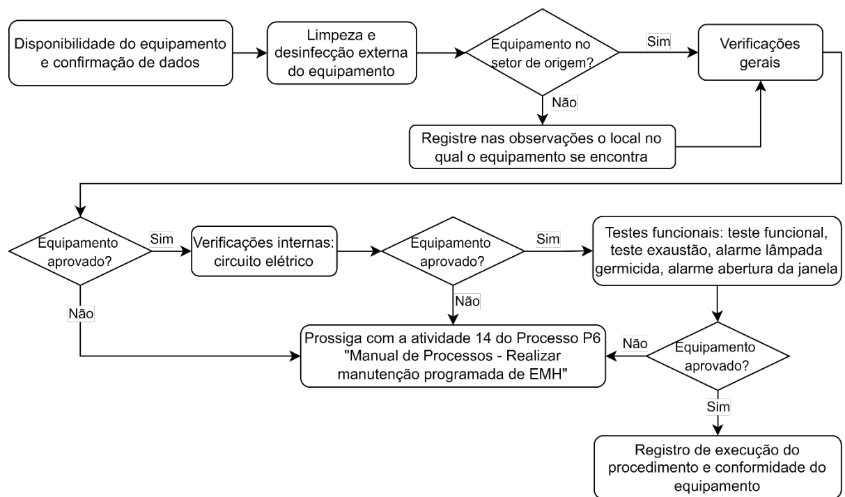
Figura 3 - Etapas de execução do procedimento de manutenção preventiva em equipamento do tipo capela de fluxo laminar.
