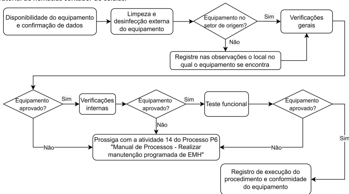
Figura 3 - Etapas de execução do procedimento de manutenção preventiva em equipamentos do tipo analisador laboratorial de hemácias contador de células.
