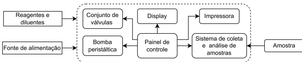
Figura 2 - Diagrama em blocos de equipamento do tipo analisador laboratorial de hemácias contador de células.
