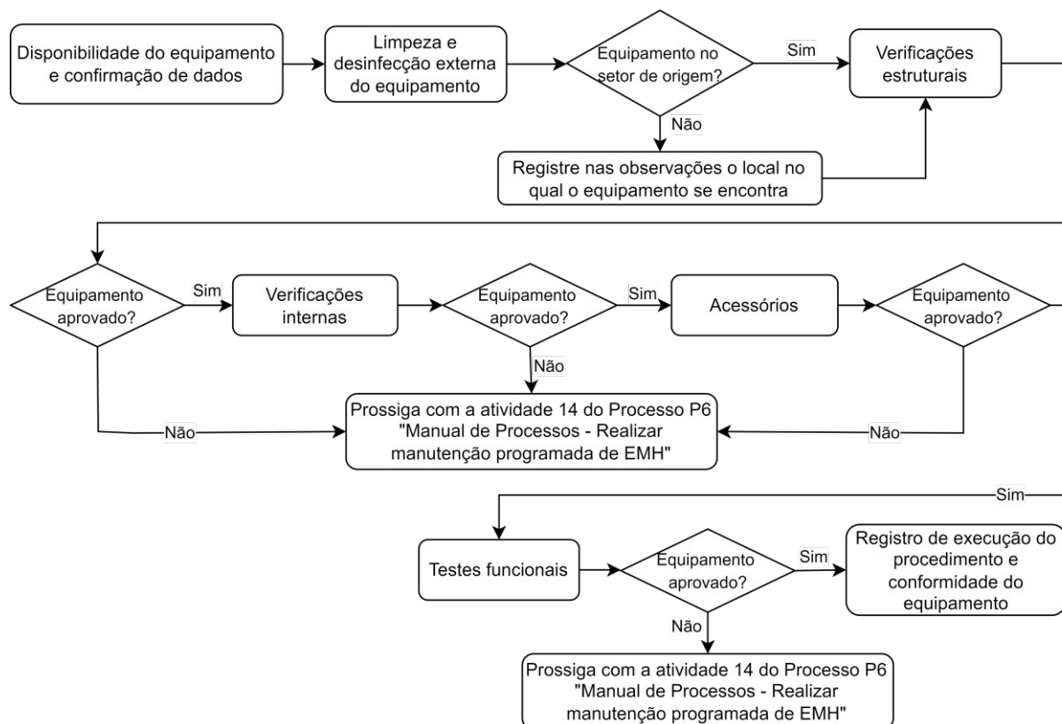
Figura 3 - Etapas de execução do procedimento de manutenção preventiva em equipamentos do tipo YAG laser.
