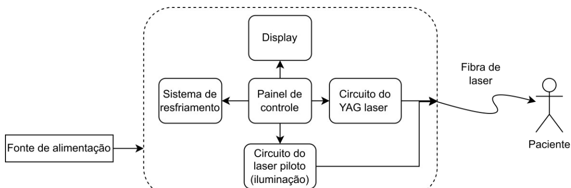
Figura 2 - Diagrama em blocos de equipamento do tipo YAG laser.
