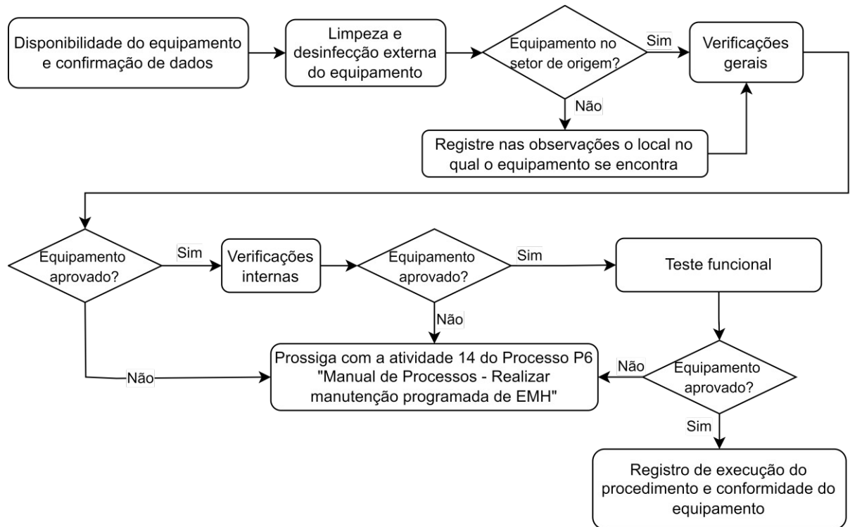
Figura 3 - Etapas de execução do procedimento de manutenção preventiva em equipamentos do tipo serra de gesso.
