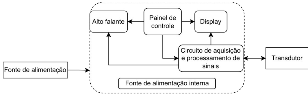
Figura 3 - Diagrama em blocos de equipamentos do tipo detector fetal.
