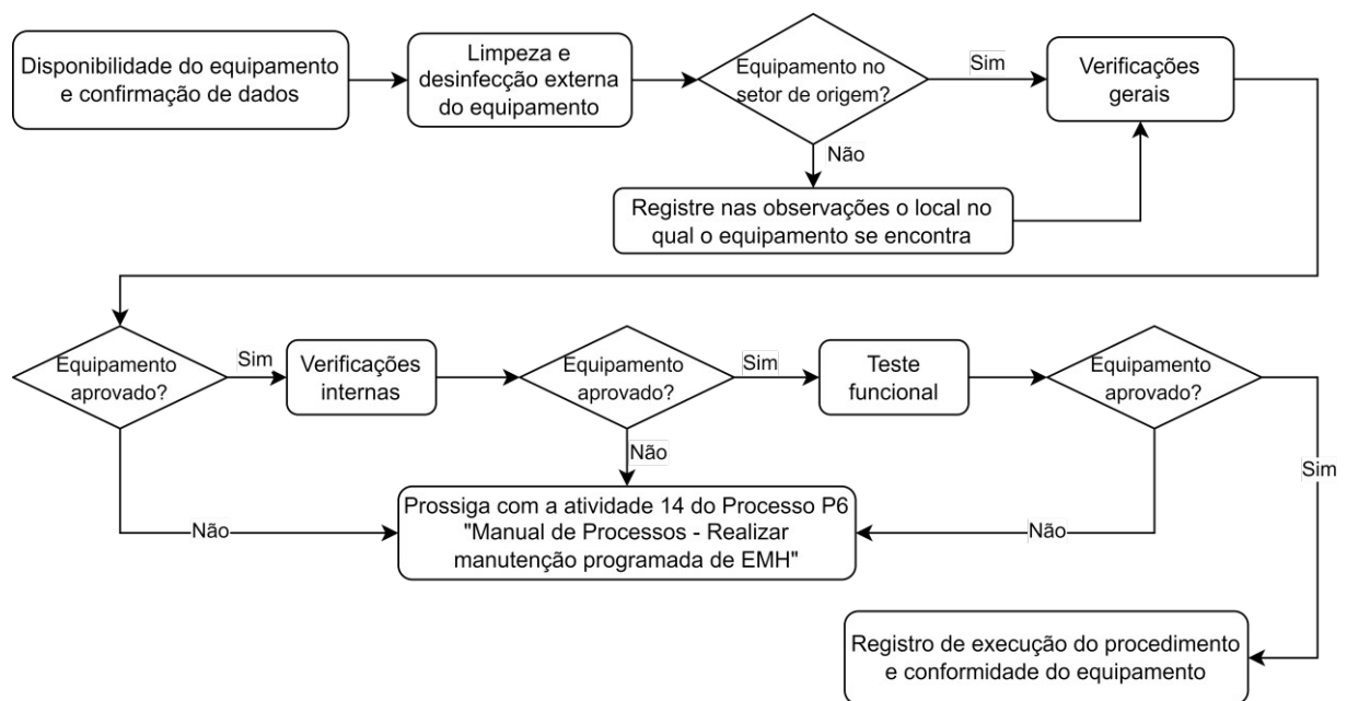
Figura 4 - Etapas de execução do procedimento de manutenção preventiva em equipamento do tipo detector fetal.
