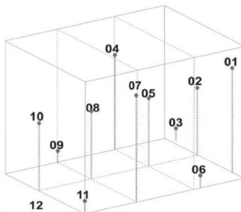
Figura 5 - Distribuição dos sensores no interior da estufa de cultura.
