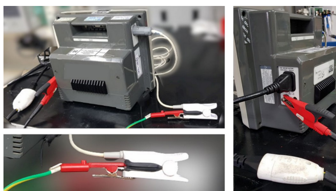
Figura 4 - Conexões de analisador de segurança elétrica à equipamento do tipo oxímetro de pulso.
