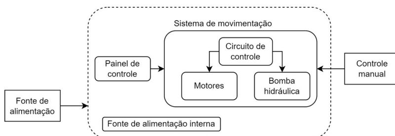
Figura 2 - Diagrama em blocos de mesa cirúrgica eletro-hidráulica.
