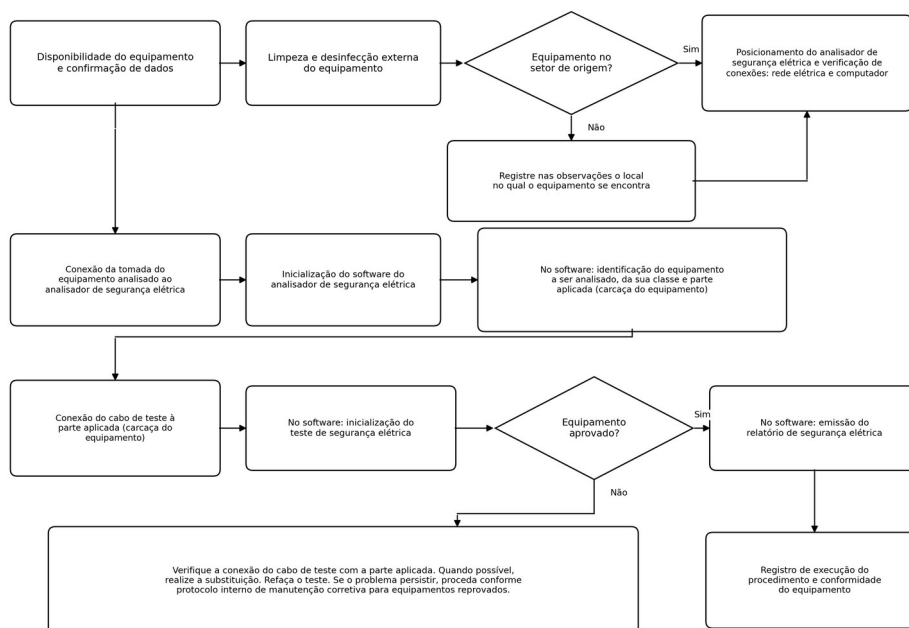
Figura 3 - Etapas de execução de teste de segurança elétrica em mesa cirúrgica.
