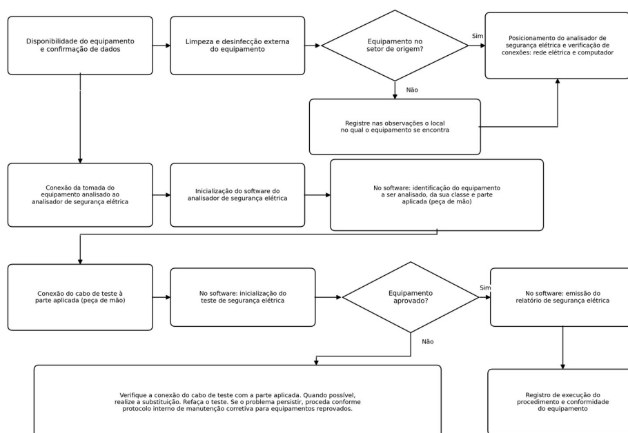
Figura 3 - Etapas de execução de teste de segurança elétrica em equipamentos do tipo facoemulsificador.
