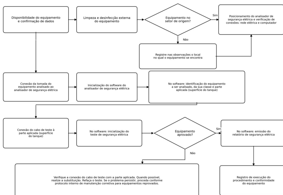
Figura 3 - Etapas de execução de teste de segurança elétrica em equipamentos do tipo banho turbilhão.
