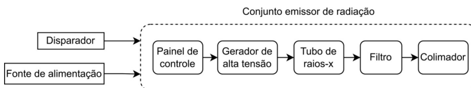
Figura 2 - Diagrama em blocos de equipamentos do tipo aparelho de raios-x odontológico.
