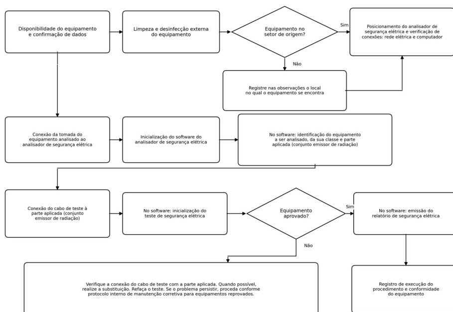
Figura 3 - Etapas de execução de teste de segurança elétrica em equipamentos do tipo aparelho de raios-x odontológico.
