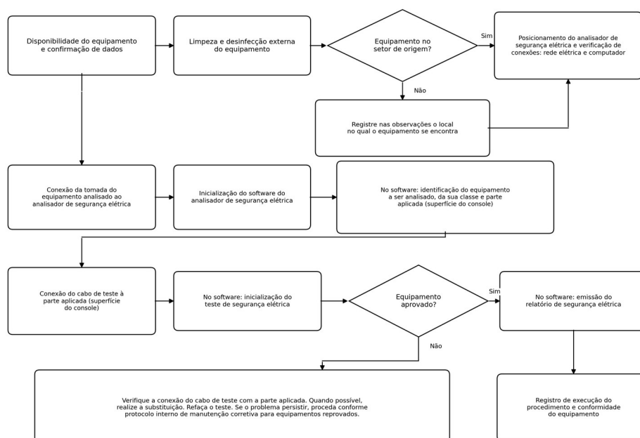
Figura 3 - Etapas de execução de teste de segurança elétrica em equipamentos do tipo injetor meio contraste.
