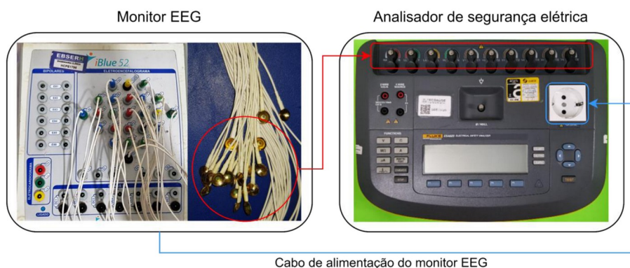
Figura 4 - Ilustração de conexões entre o monitor EEG e o analisador de segurança elétrica.
