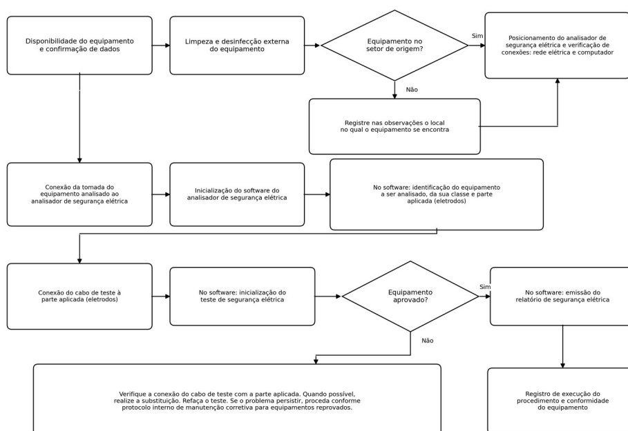
Figura 3 - Etapas de execução do procedimento de segurança elétrica em equipamentos do tipo monitor EEG.
