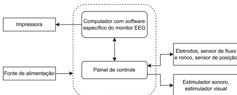
Figura 2 - Diagrama em blocos de equipamento do tipo monitor EEG.
