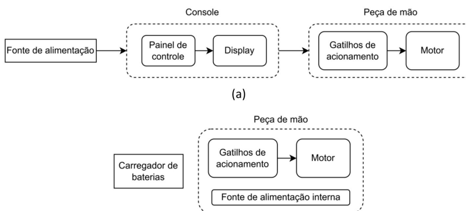
Figura 1 - Diagrama em blocos de equipamentos do tipo perfurador cirúrgico elétrico com console (a) e à bateria (b).
