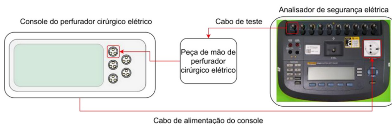
Figura 4 - Indicação de conexões entre perfurador cirúrgico elétrico e analisador de segurança elétrica.
