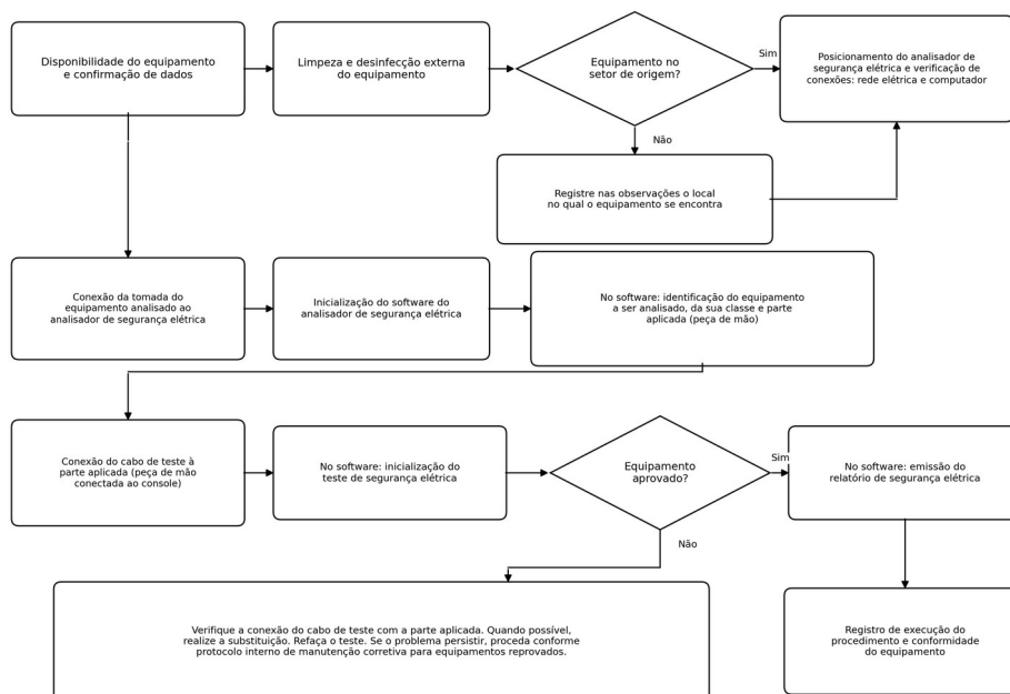
Figura 3 - Etapas de execução de teste de segurança elétrica em equipamentos do tipo perfurador cirúrgico elétrico.
