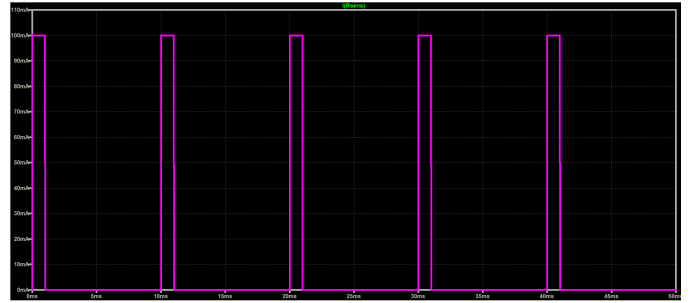
Figura 10. Corriente de excitación pulsada con un ciclo de trabajo del 10%.
