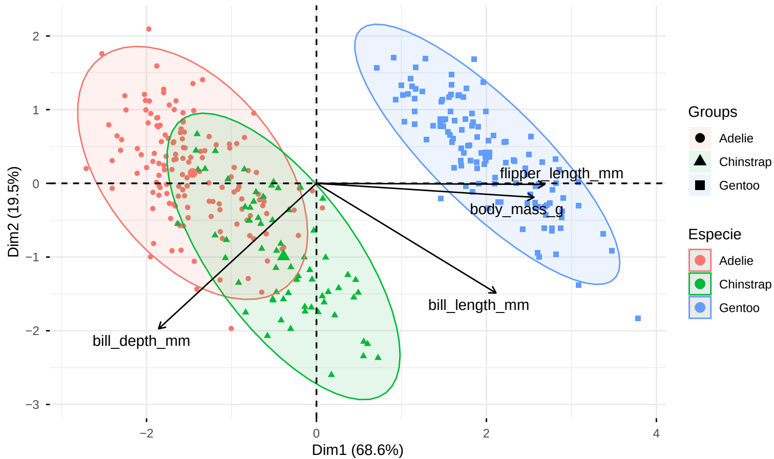
Biplot del PCA de Penguins
