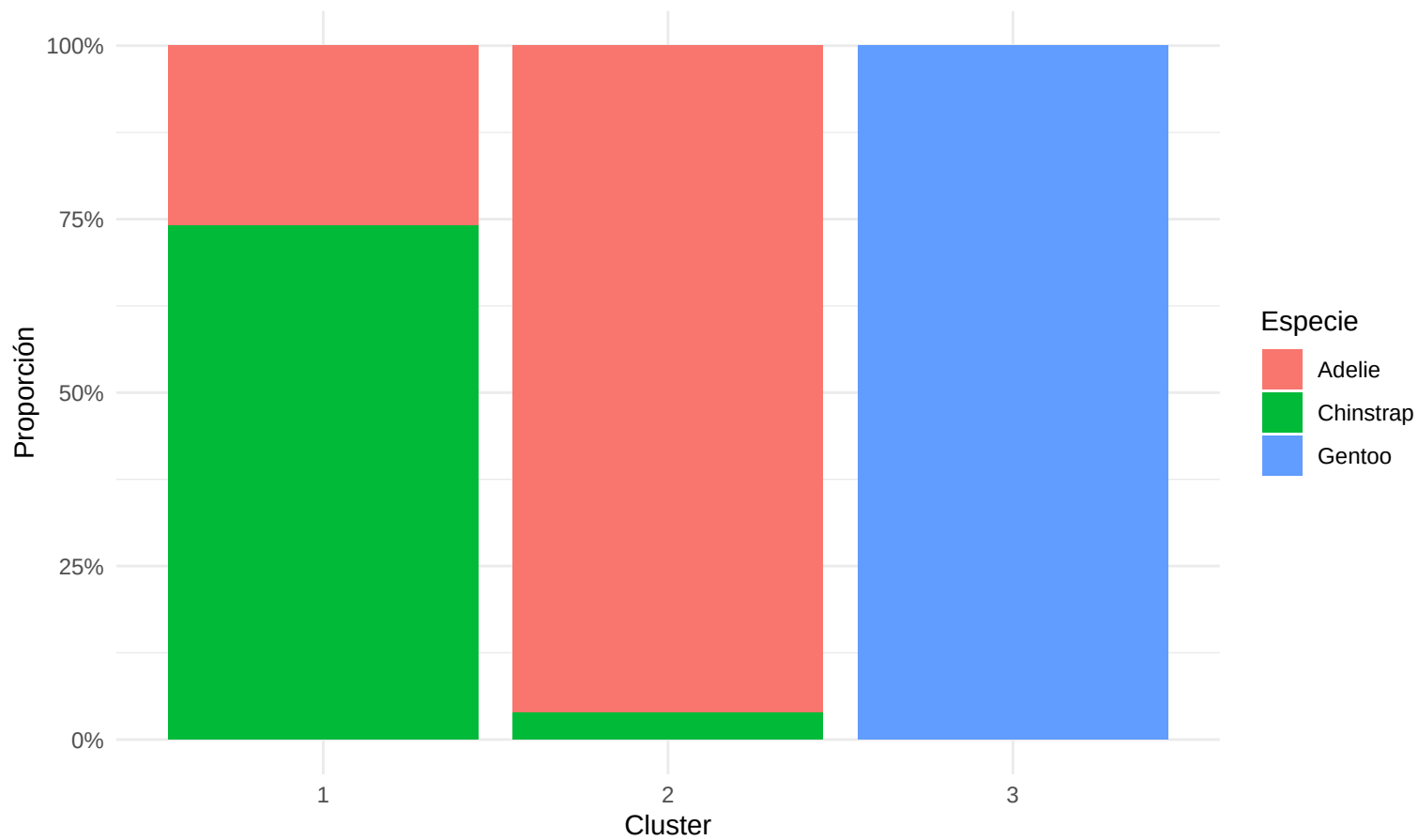
Composición de especies en cada cluster
