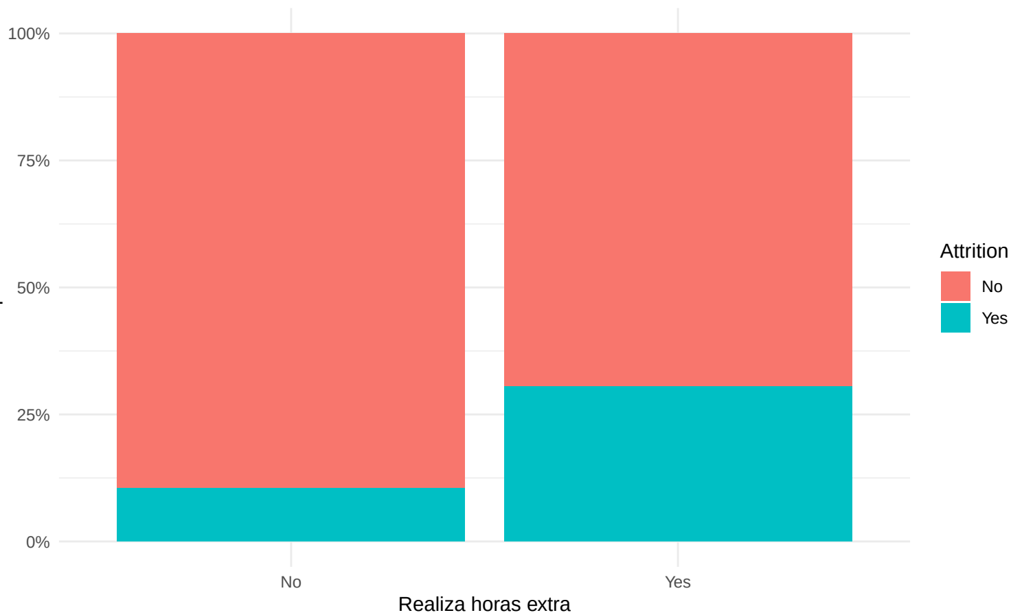
Proporción de rotación laboral según horas extra
