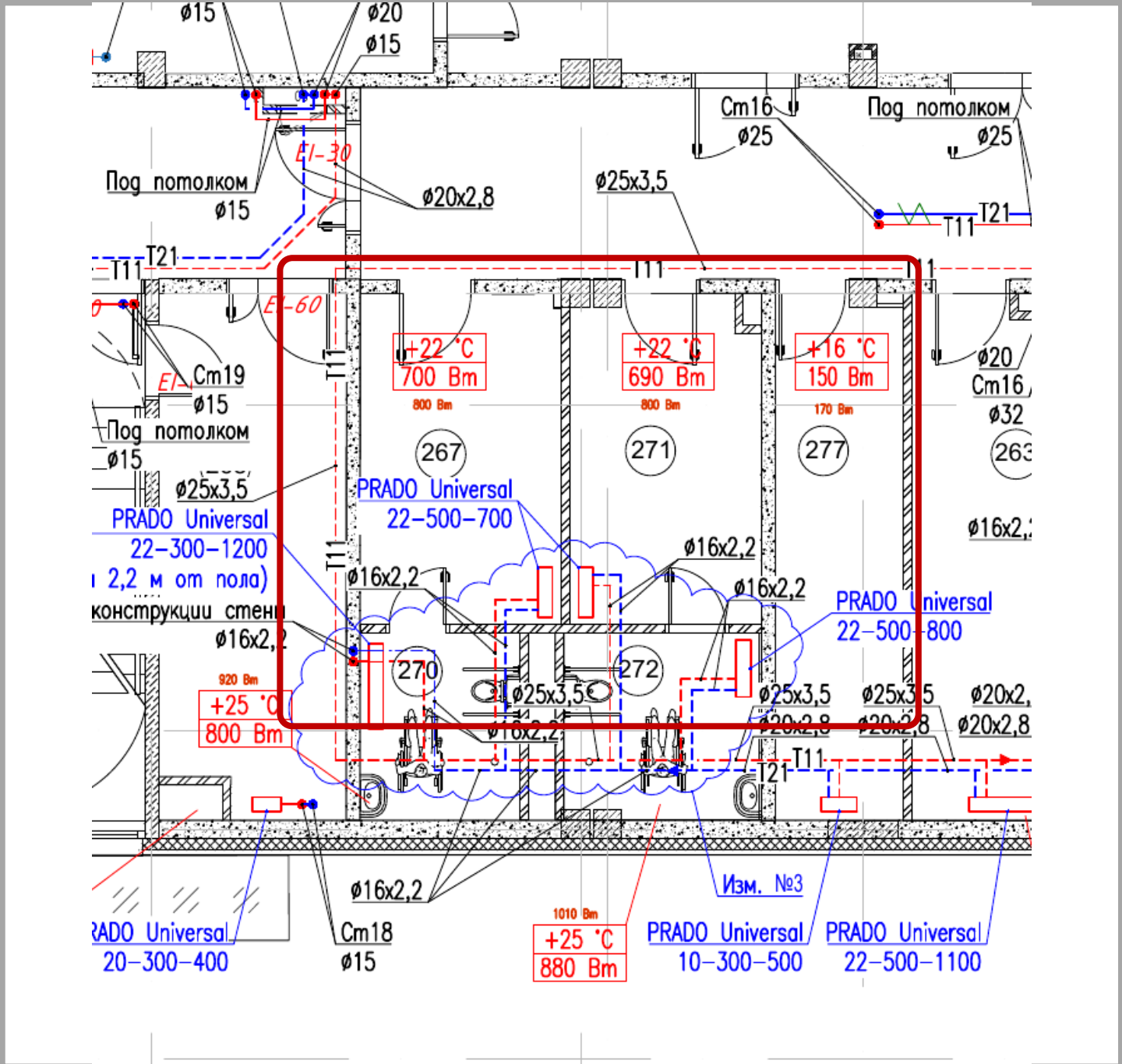
Показаны отопительные приборы и разводка; условные обозначения контуров теплого пола отсутствуют.
