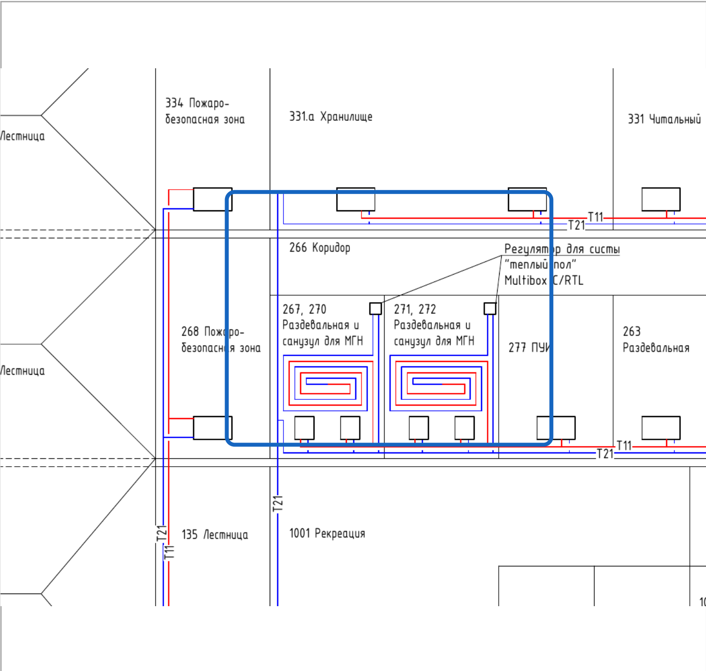
В помещениях 267/270 и 271/272 показаны два самостоятельных контура теплого пола.
