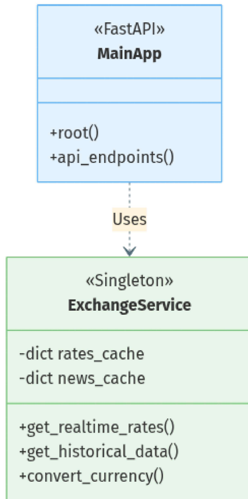
图 2: ExchangeService 类结构
