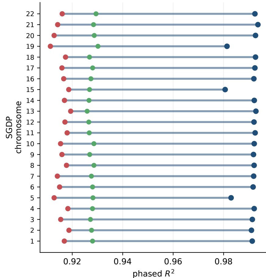
(d) 5% masked
