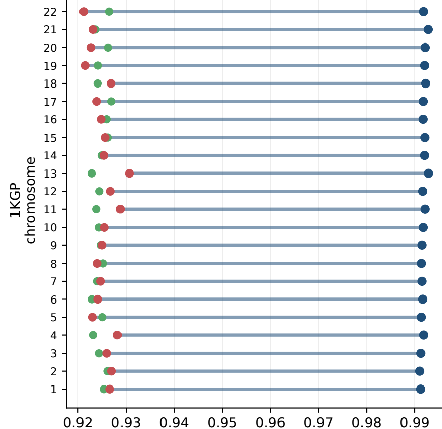
(d) 5% masked
