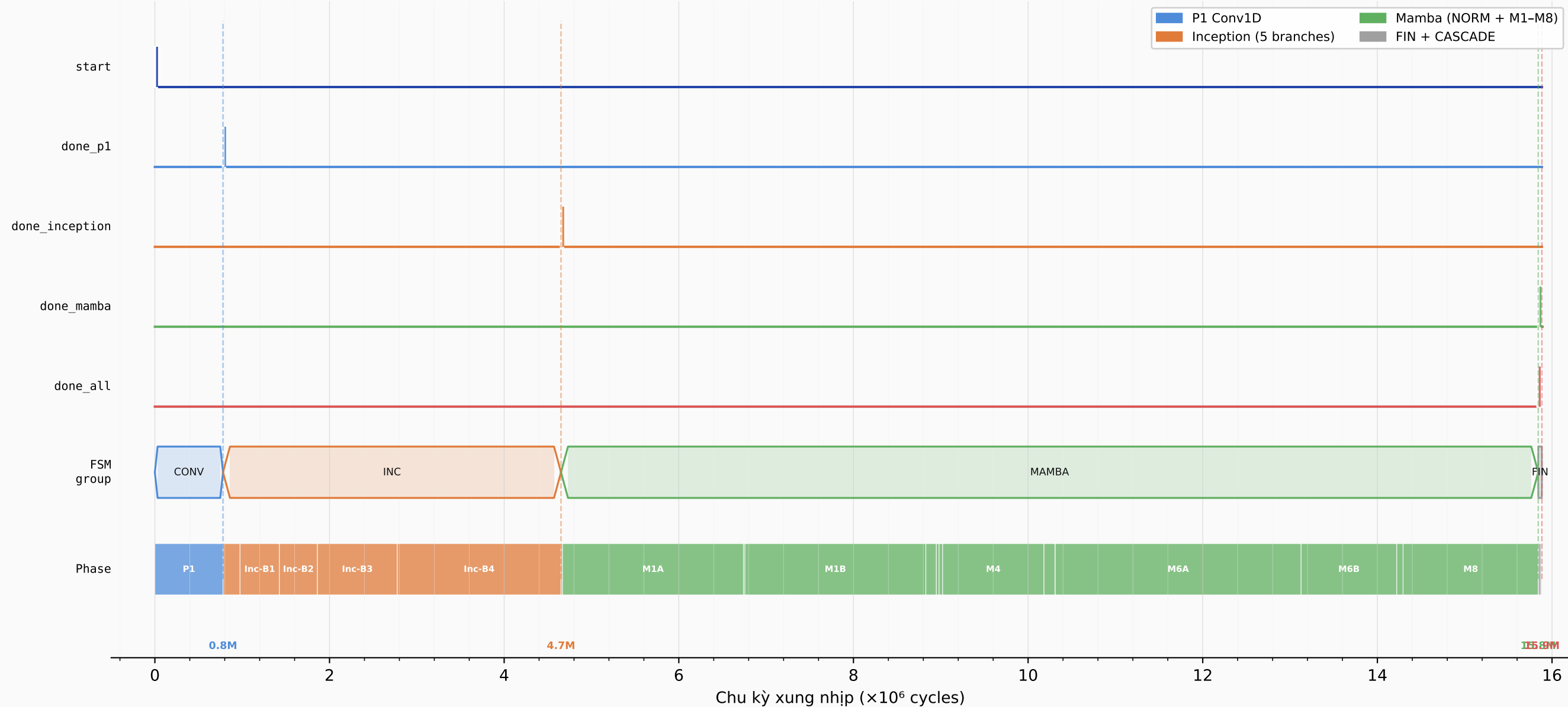
Hình 4.1 — Dạng sóng FSM một khối ITM (Block 0, T=1000) Tổng \approx 15.9\text{M} chu kỳ | Fmax = 108.2 MHz | Latency \approx 147 ms
