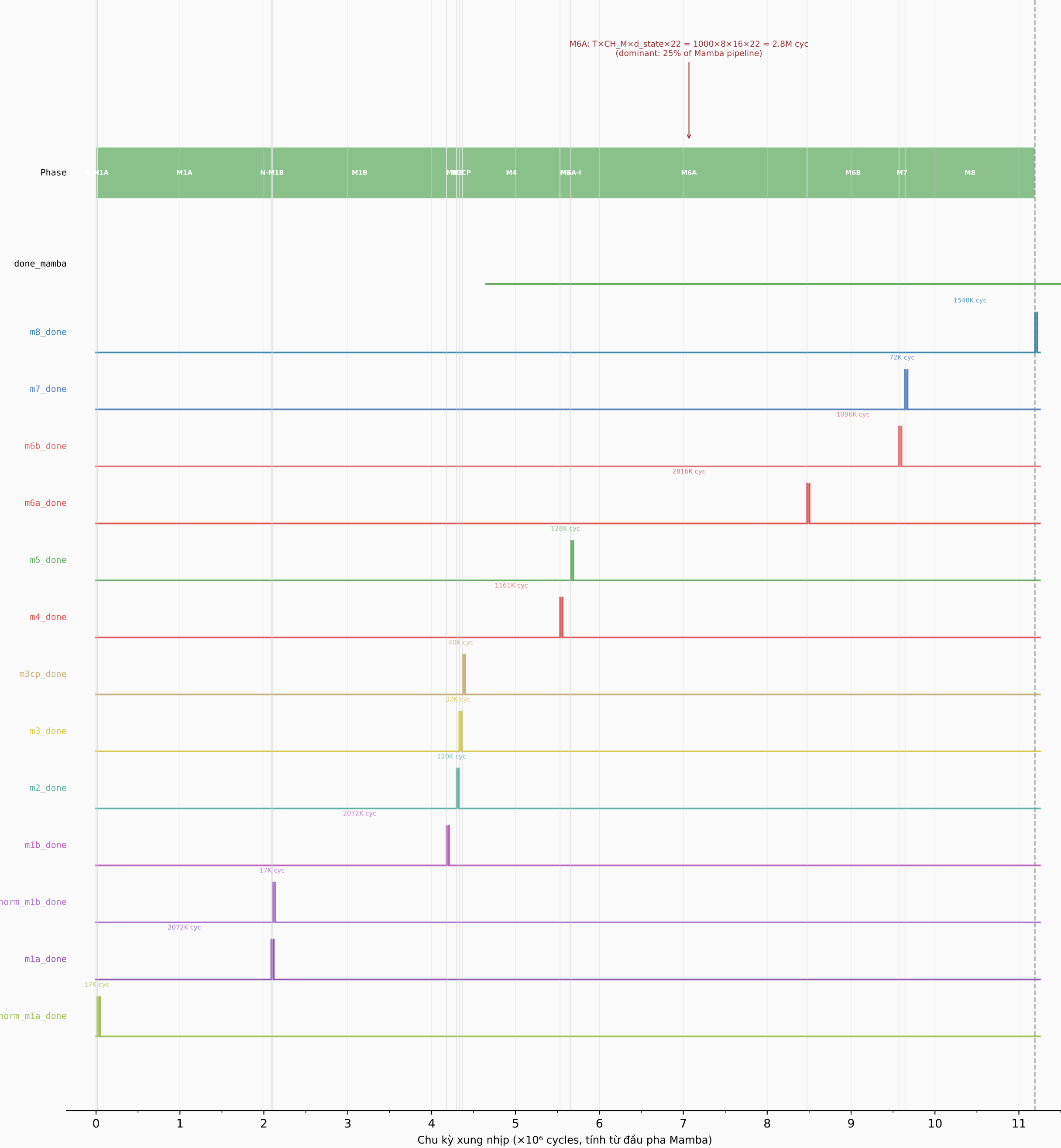
Hình 4.2 — Dạng sóng FSM pha Mamba M1-M8 (Block 0, T=1000) Mamba pipeline ≈ 11.2M chu kỳ | Chiếm 70% tổng latency khối
