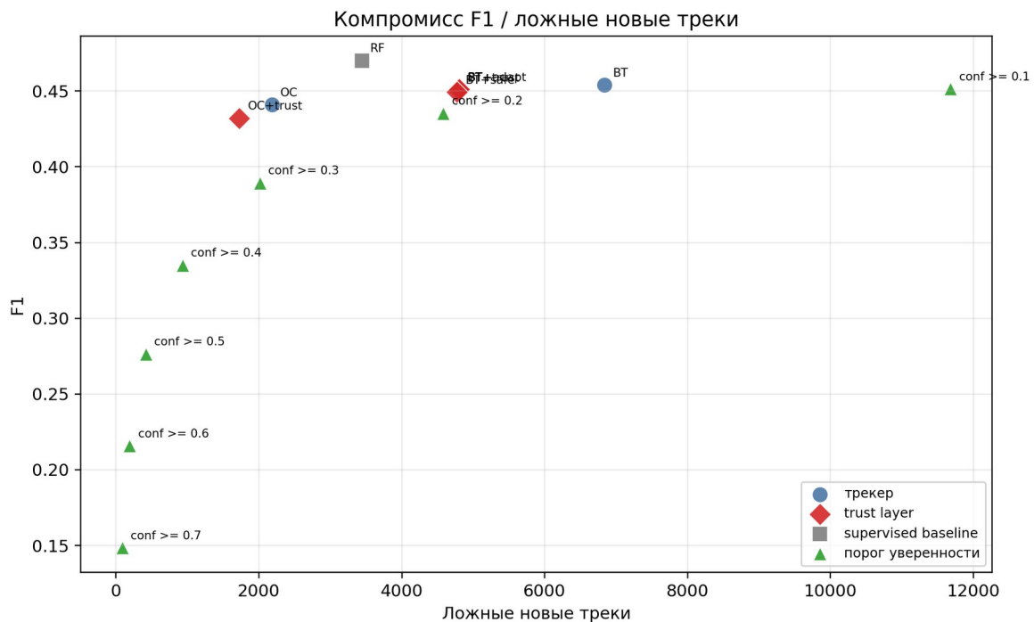
Рис. X. Компромисс между F1 и числом ложных новых треков на VisDrone YOLOv8s. Доверительный слой не максимизирует F1 любой ценой, а выбирает более осторожную рабочую точку, где в карту попадает меньше ложных новых треков. Контрольные точки с фиксированным порогом уверенности показывают, какая часть эффекта связана с подавлением низкоуверенных кандидатов.
