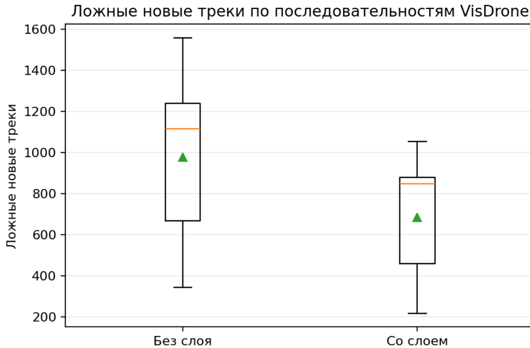
Рисунок. Распределение числа ложных новых треков по последовательностям VisDrone. Доверительный слой снижает величину эффекта, но Holm-corrected significance не достигается.
