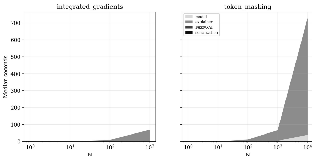
Рисунок 4.27 — Декомпозиция полного времени по этапам конвейера
