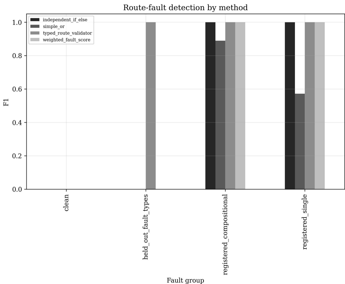
Рисунок 4.26 — Качество обнаружения нарушений для четырёх проверяющих схем
