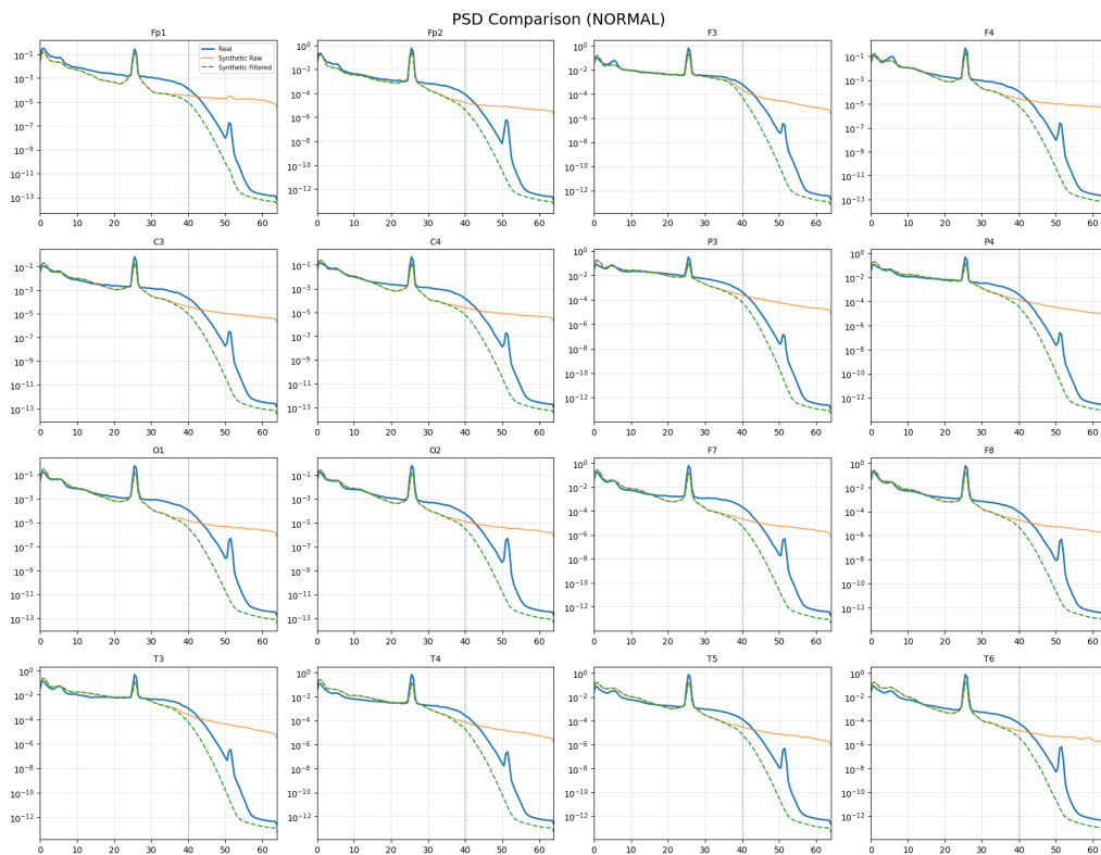
Gambar 4.2. Visualisasi Domain Frekuensi Sampel Sinyal EEG Sintetis
