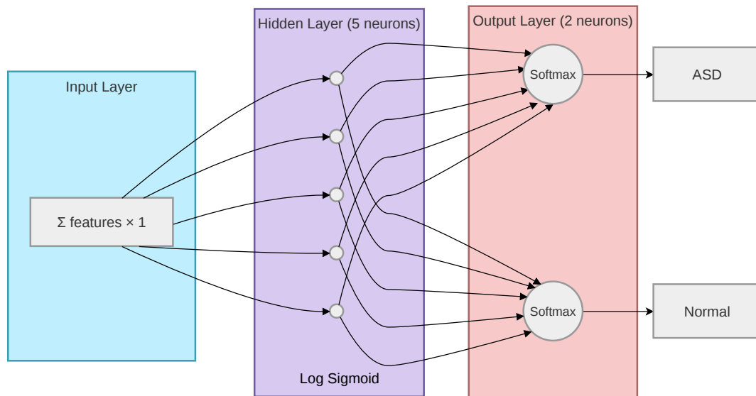
Gambar 3.9. Arsitektur model Deep Neural Network (DNN) yang digunakan dalam penelitian
