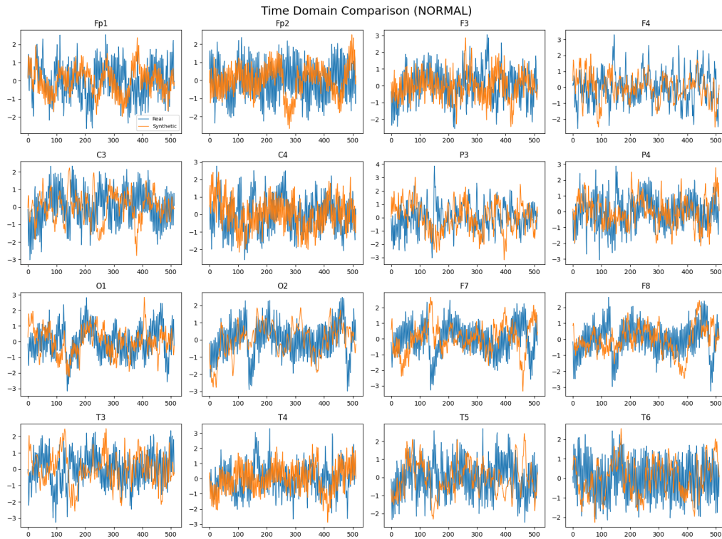
Gambar 4.1. Visualisasi Domain Waktu Sampel Sinyal EEG Sintetis
