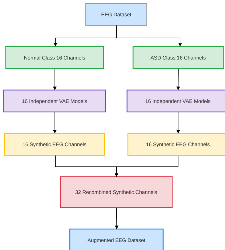
Gambar 3.8. Diagram aliran generasi data sintesis
