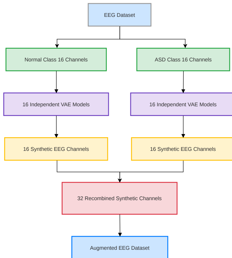
Gambar 3.8. Diagram aliran generasi data sintetis
