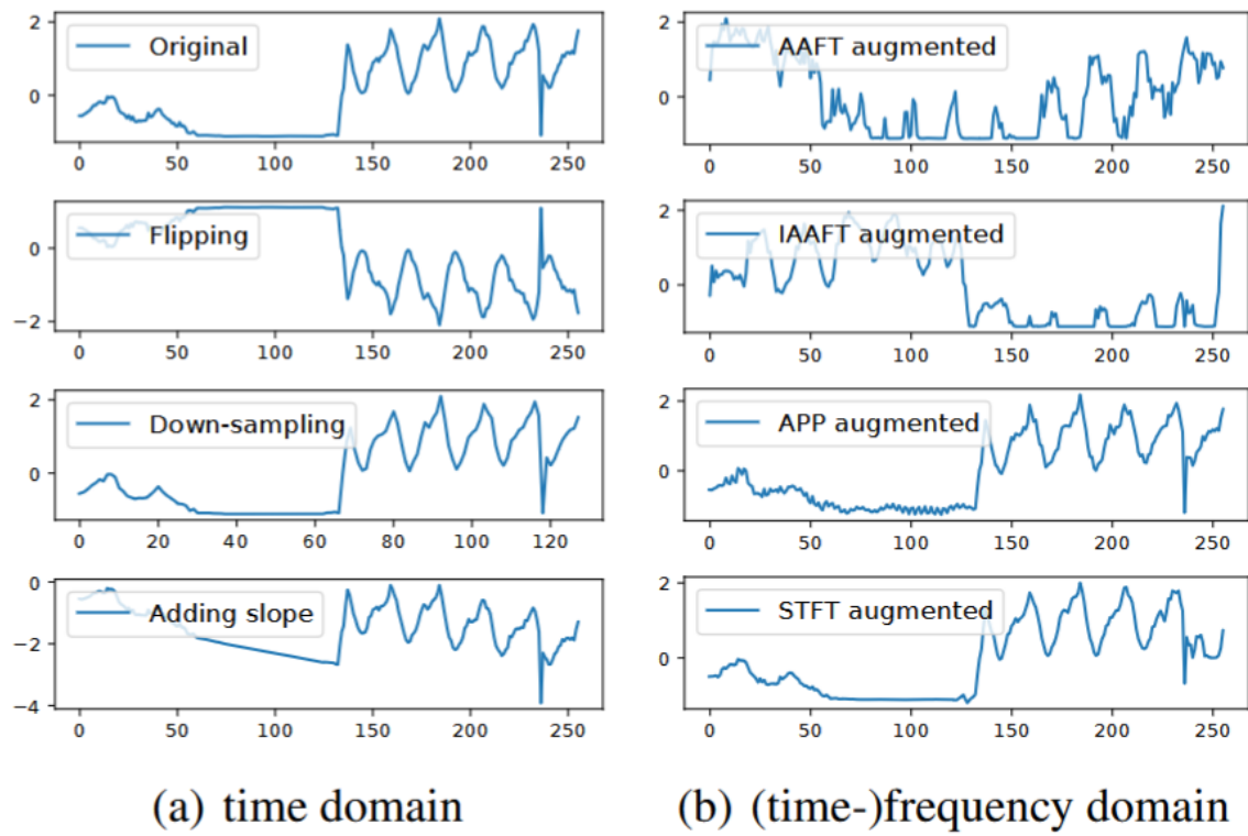
Gambar 2.7. Ilustrasi metode augmentasi pada data time-series
