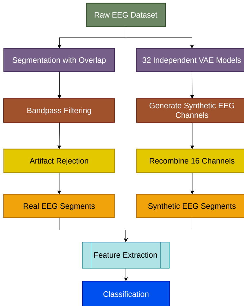
Gambar 3.9. Diagram alur integrasi data sintetis pada proses klasifikasi
