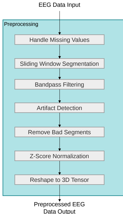
Gambar 3.2. Diagram aliran proses prapemrosesan sistem
