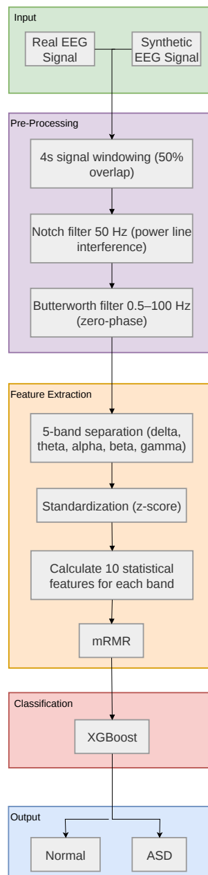
Gambar 3.4. Diagram model klasifikasi
