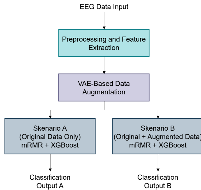
Gambar 3.1. Diagram aliran data pada sistem
