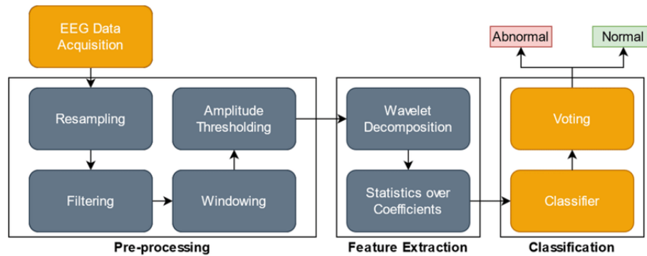
Gambar 2.6. Ilustrasi umum pipeline klasifikasi ASD berbasis sinyal EEG
