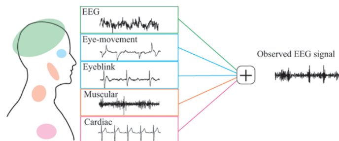
Gambar 2.4. Bentuk-Bentuk artefak pada sinyal EEG
