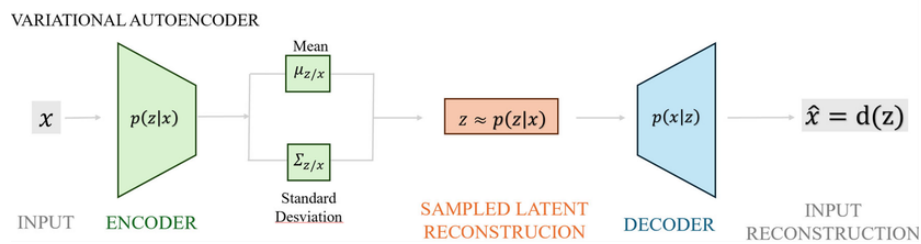
Gambar 2.8. Arsitektur umum Variational Autoencoder (VAE)
