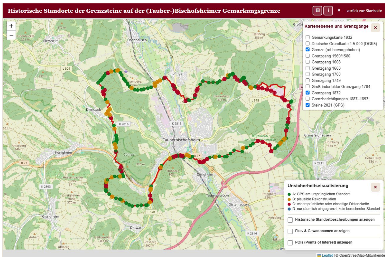
Abb. 4: Karte der Grenzsteine, hier mit der Ebene „Grenzgang 1872“: grün eingemessene Steine, orange und rot berechnete Standorte verschwundener Steine mit Sicherheitsklasse
