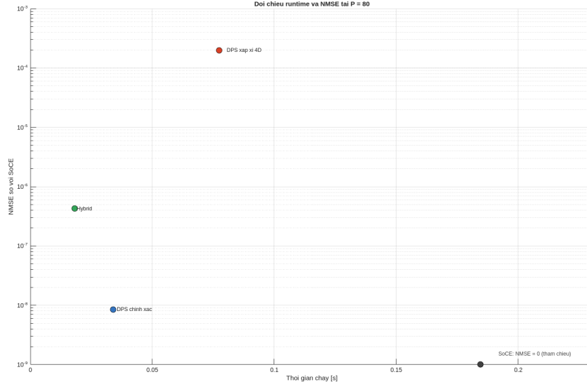
Hình 4.6 Biểu đồ runtime–NMSE của bốn nhánh tại P = 80
