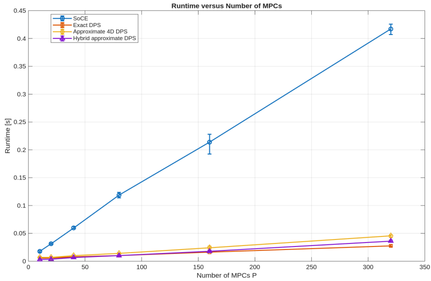
Hình 4.5 Thời gian chạy của SoCE, DPS chính xác, DPS xấp xỉ 4D và phương pháp hybrid khi thay đổi số MPC
