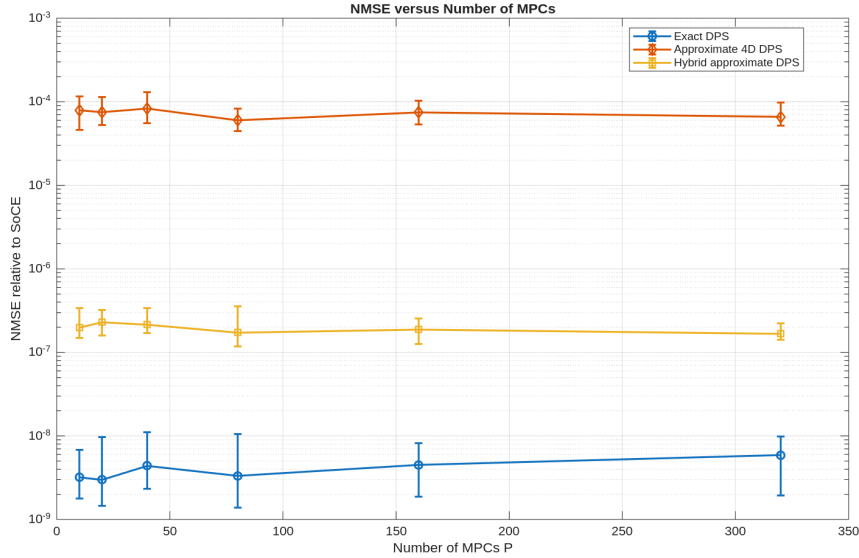
Hình 4.4 NMSE của DPS chính xác, DPS xấp xỉ 4D và phương pháp hybrid khi thay đổi số MPC
