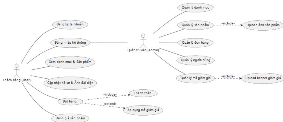
Hình 2.1: Sơ đồ Usecase diagram
