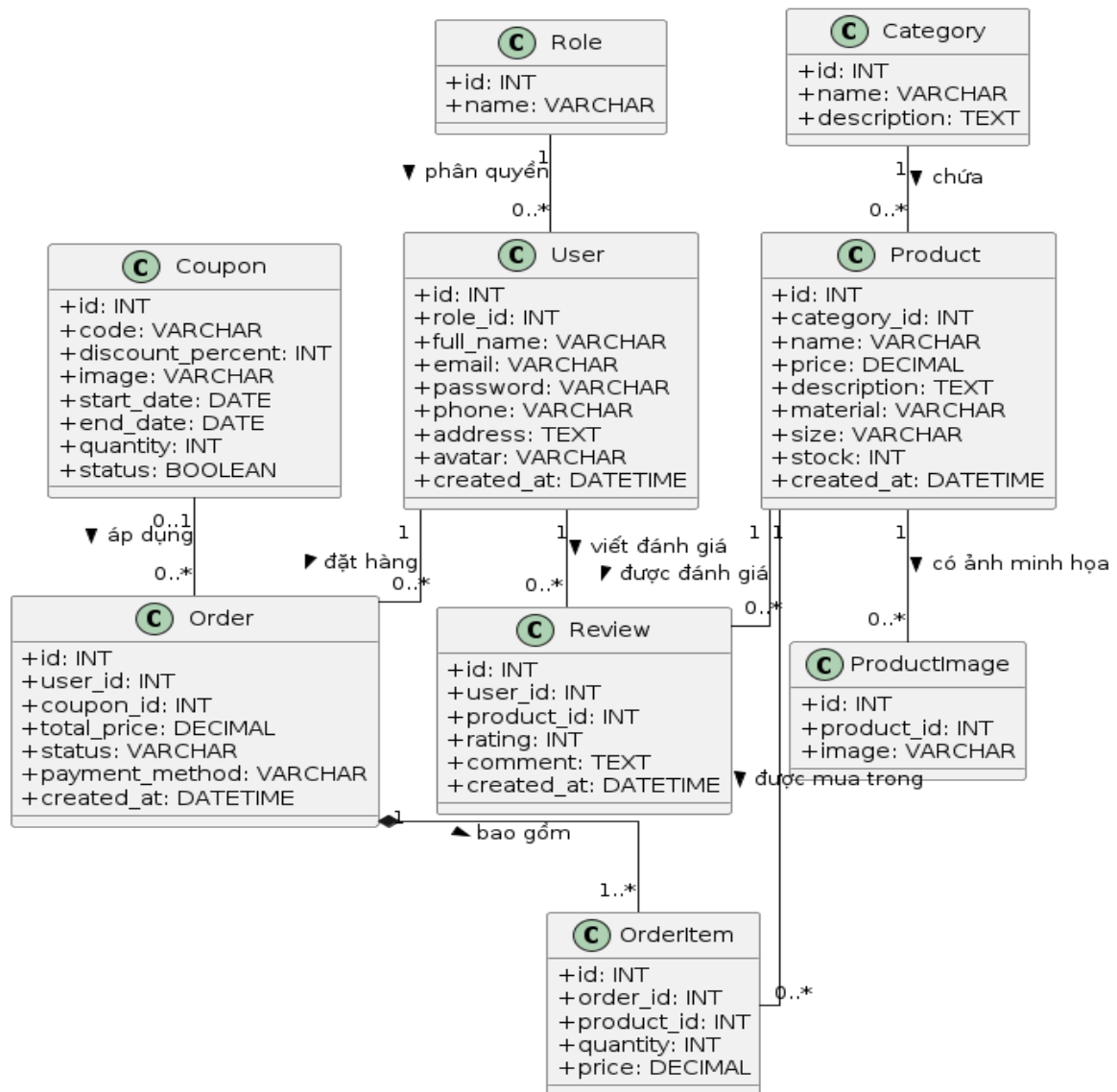
Hình 2.2: Sơ đồ Class diagram
