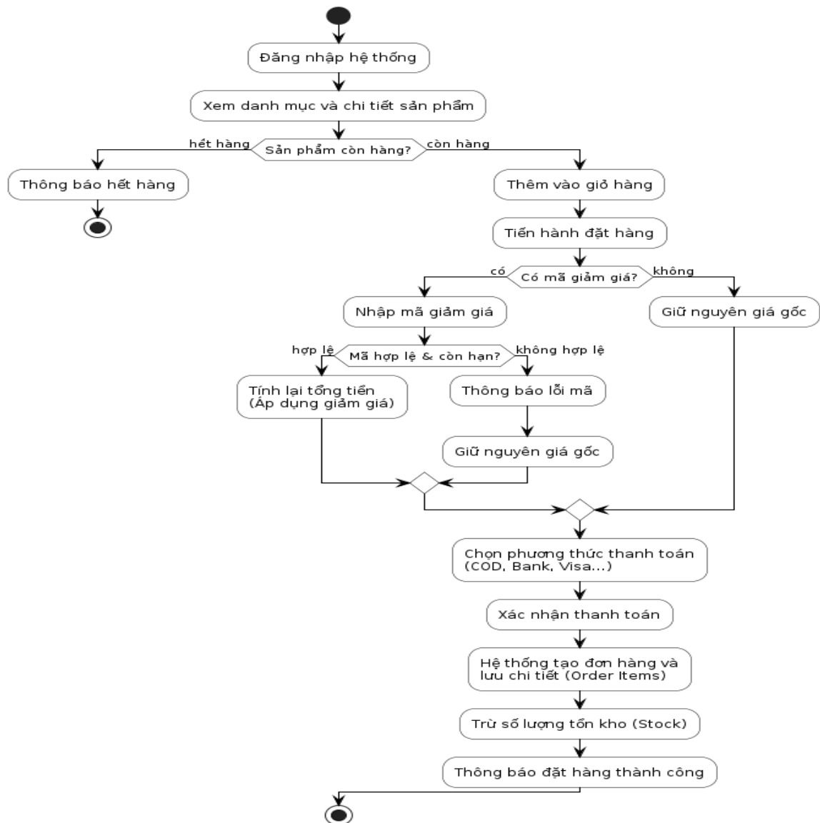
Hình 2.3: Sơ đồ Activity diagram
