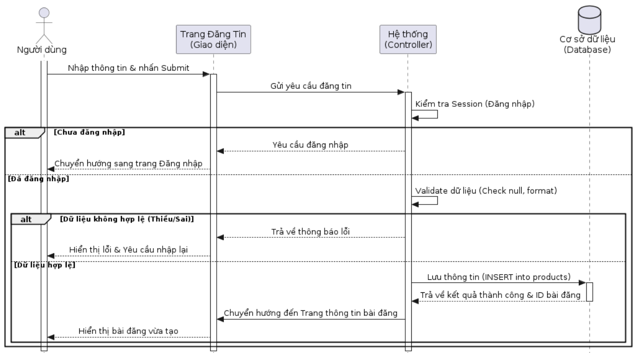
Hình 2.4: Sơ đồ Sequence diagram
