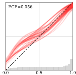
BICR (Ours)
