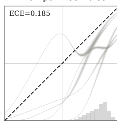
Prompt Ensembles
