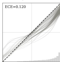
SAPLMA
