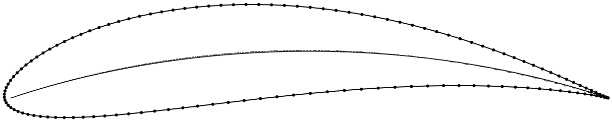
Figure 15: Medial axis of the VON KÁRMÁN–TREFFTZ airfoil
