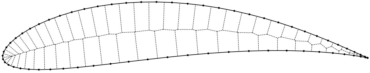
Figure 7: VORONOI diagram of the VON KÁRMÁN–TREFFTZ airfoil
