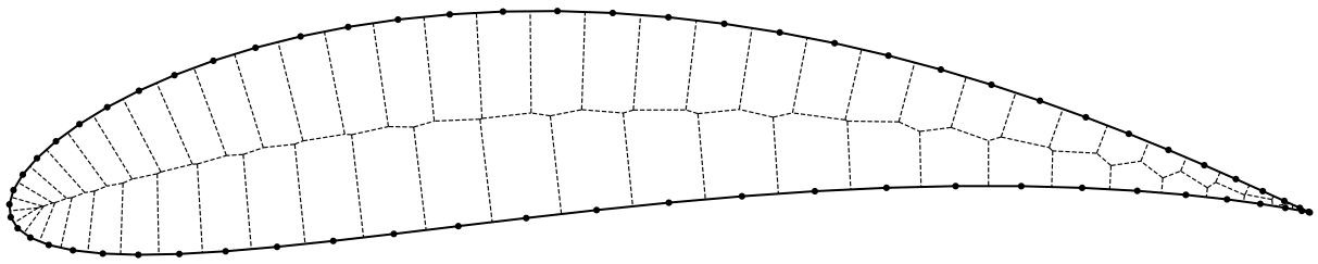
Figure 21: VORONOI diagram of the VON KÁRMÁN–TREFFTZ airfoil
