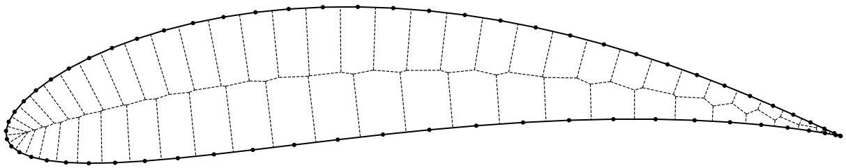
Figure 12: VORONOI diagram of the VON KÁRMÁN-TREFFTZ airfoil
