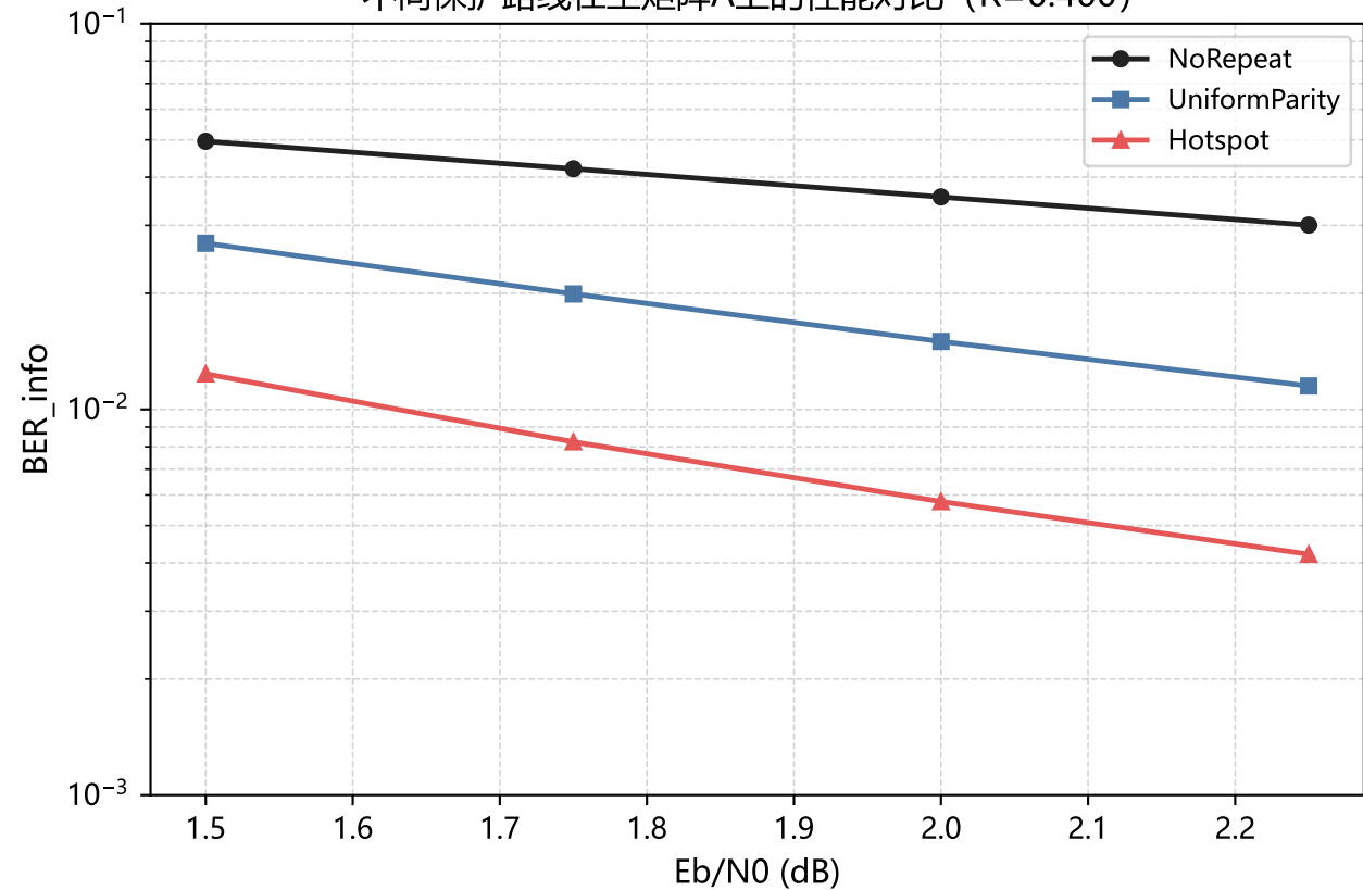
不同保护路线在主矩阵A上的性能对比 (R=0.400)
