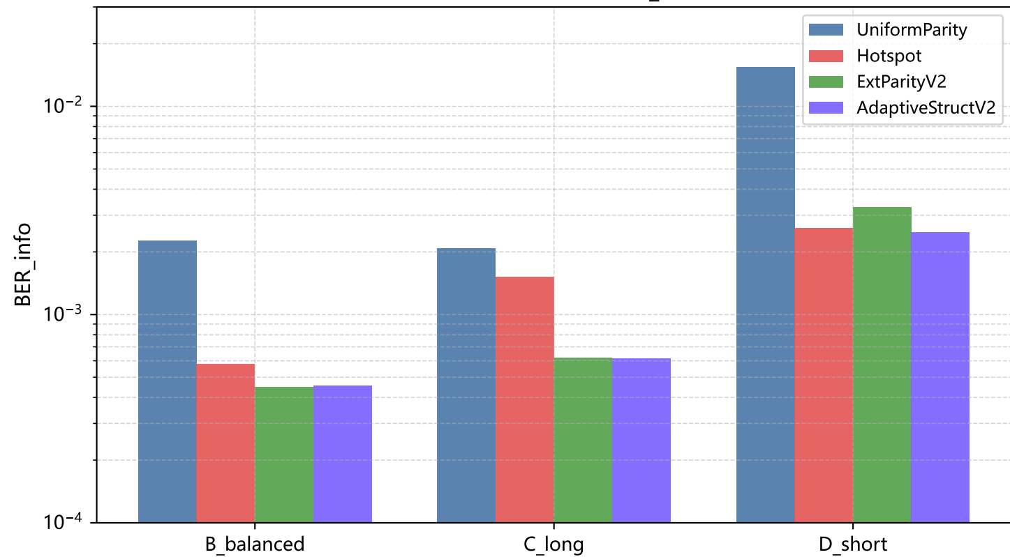
多矩阵泛化中不同方法的BER_info对比
