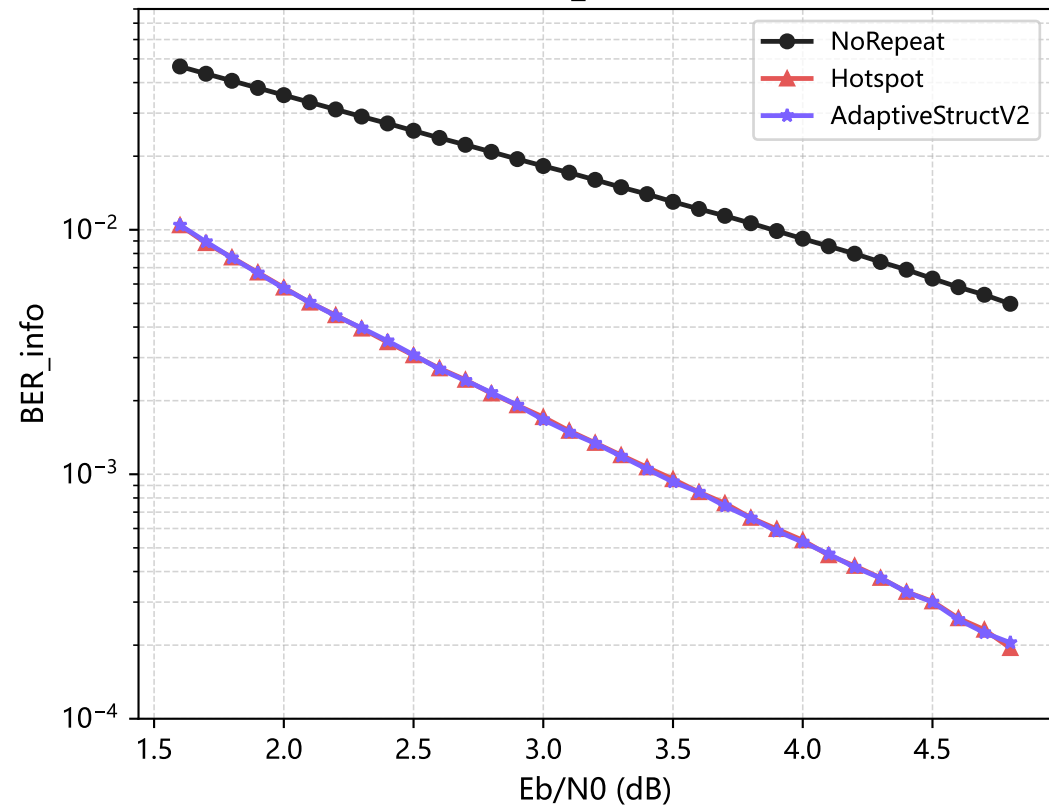
阈值扫描：BER_info随Eb/N0变化
