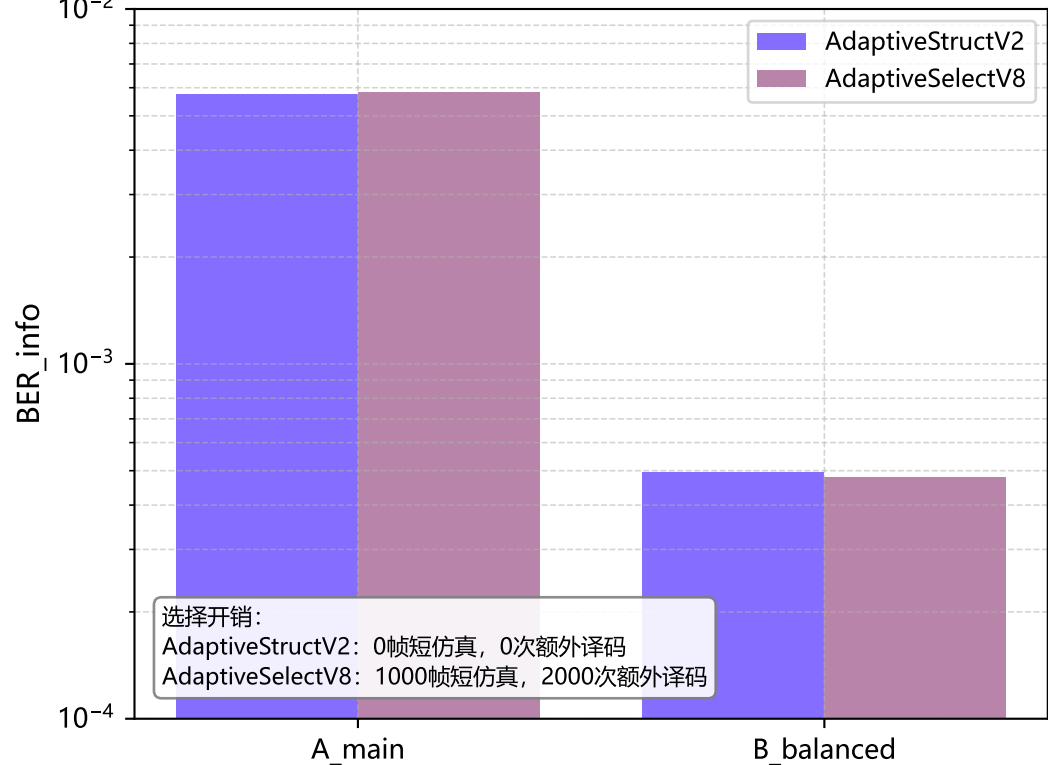
工程化选择对比 ( E_b/N_0=2.0 dB)
